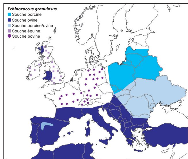
FIGURE 1. Répartition de l'espèce Echinococcus granulosus en Europe.
