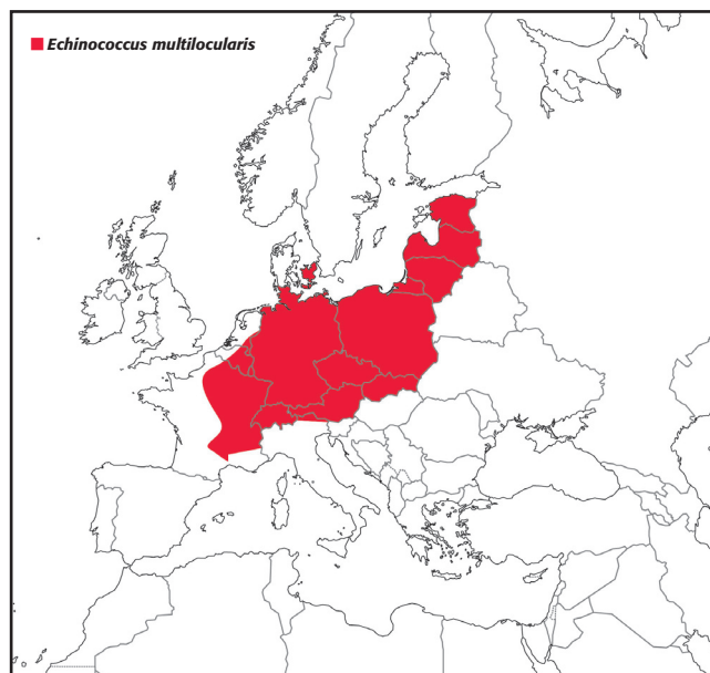
FIGURE 2. Répartition de l'espèce Echinococcus multilocularis en Europe
